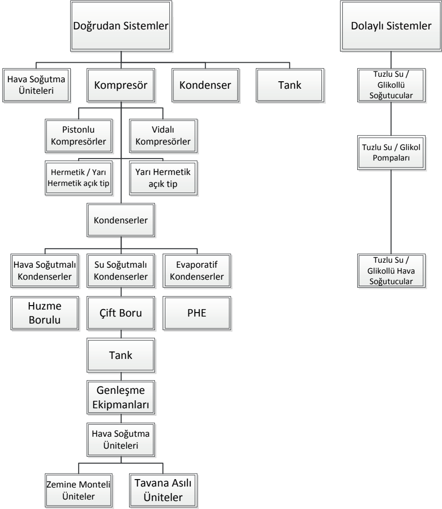
Şekil 3.1: HCFC/HFC ile çalışan sistemlerin temel bileşenleri.
